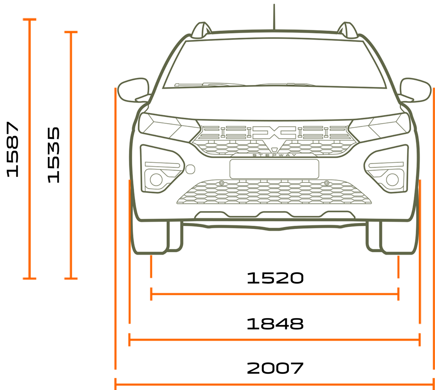
IŠ PRIEKIO
