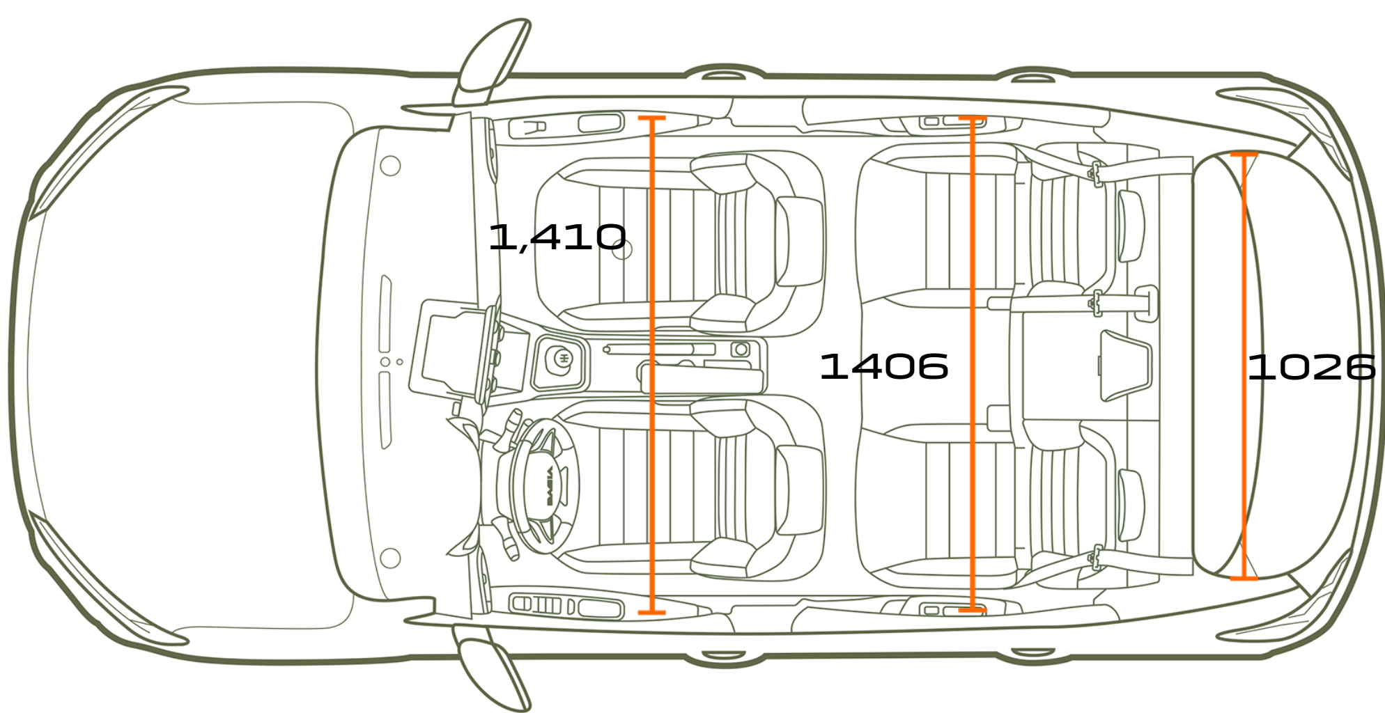
IŠ VIRŠAUS
