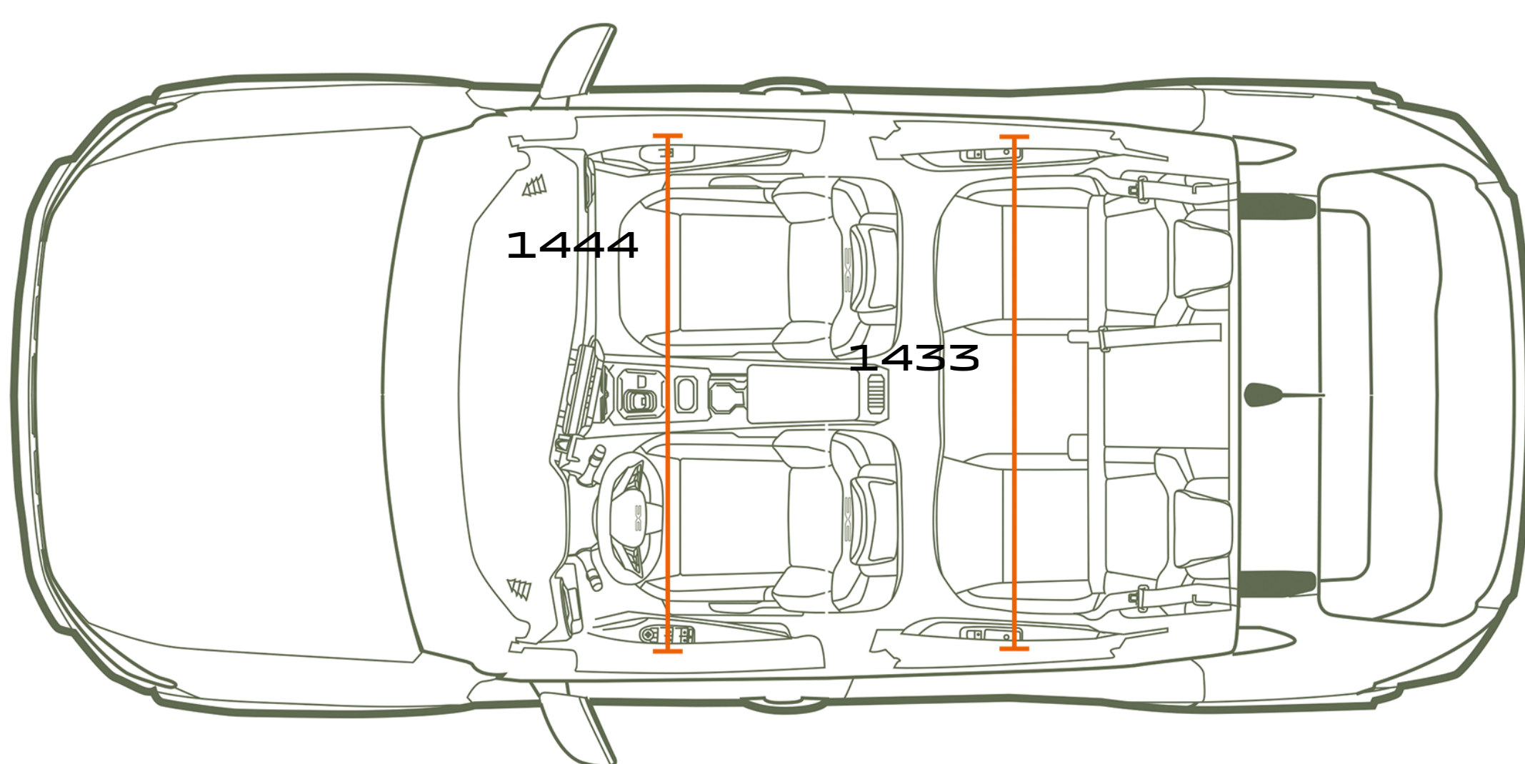
IŠ VIRŠAUS
